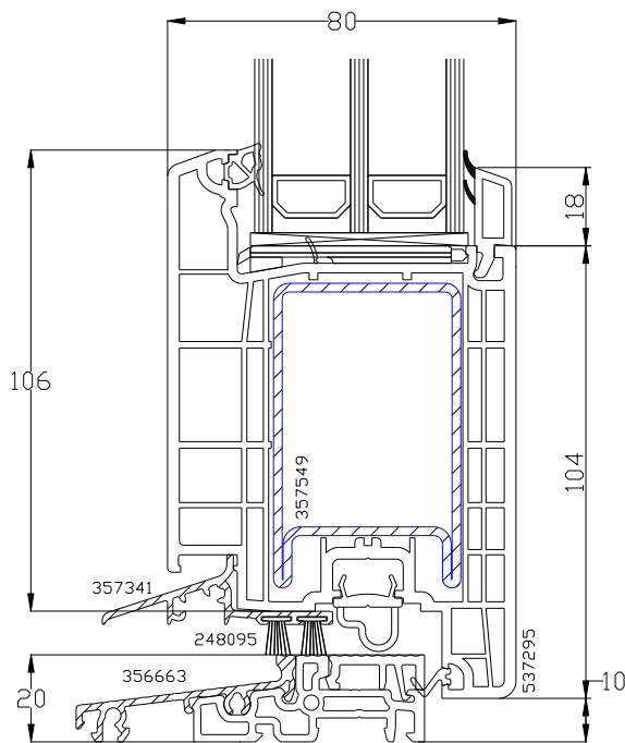
Schwelle 356663 + Flügel 537295
