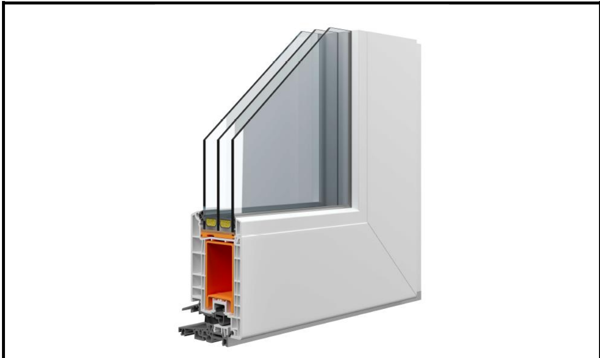
Schwelle 356663 + Flügel 537295
