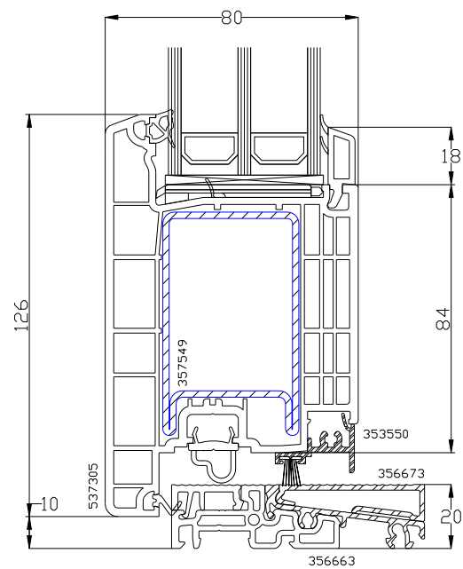
Schwelle 356663 + Flügel 537305
