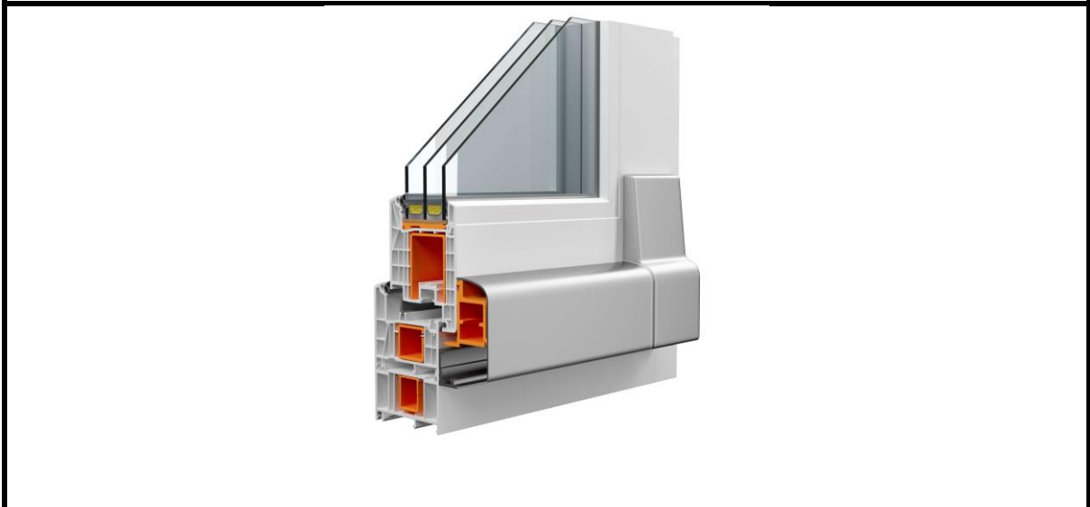
Rahmen 537675 + Flügel 537565 + Verbreiterung 45 PSK-Z (SIEGENIA)
