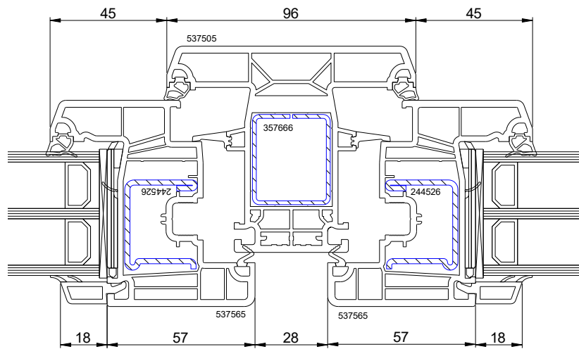
Flügel 2x537675 + Pfosten 537515
