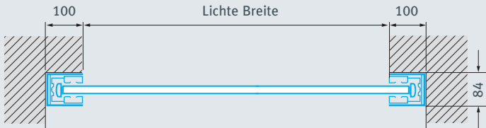
Platzbedarf bei Montage in der Leibung
