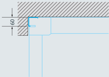
Sturzblende bei Garage ohne Sturz
