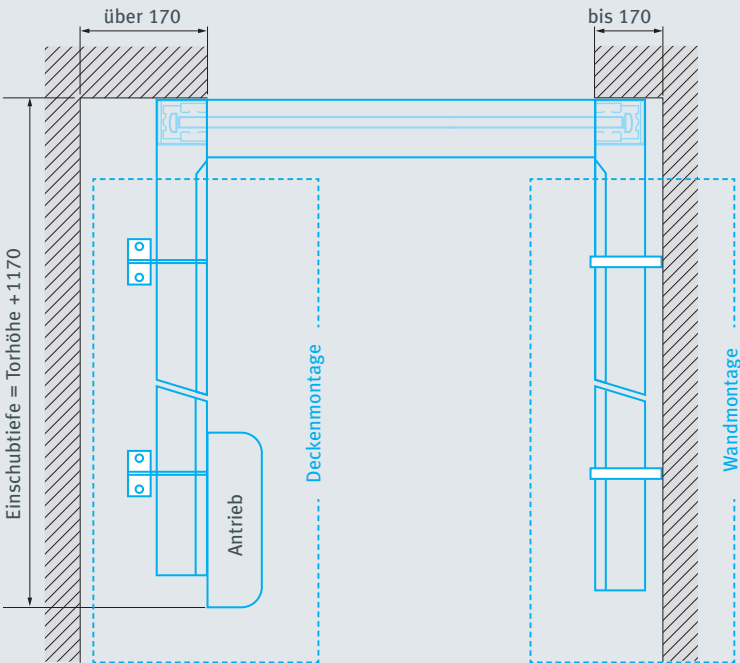
Befestigung der horizontalen Führungsschienen
